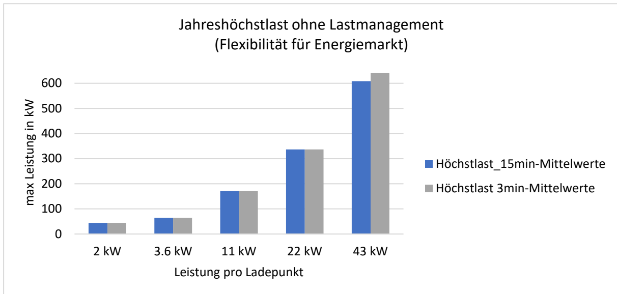
Abbildung 6: Jahreshöchstlast bei Strategie „Flexibilität für Energiemarkt“ mit Lastmanagement
