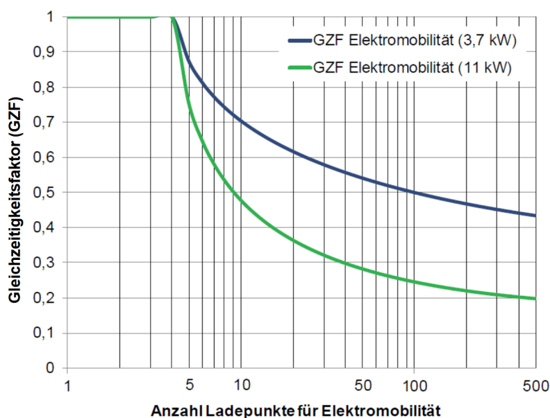
Abbildung 1: Der Gleichzeitigkeitsfaktor für Ladeinfrastruktur im privaten (nichtöffentlichen) Raum für ungesteuertes Laden, Quelle (VBEW, 2018)
