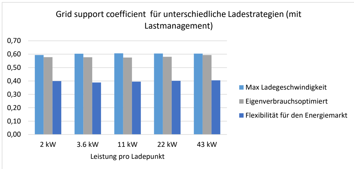
Abbildung 12: Grid support coefficient für die verschiedenen Ladestrategien und Ladeleistungen (mit Lastmanagement)
