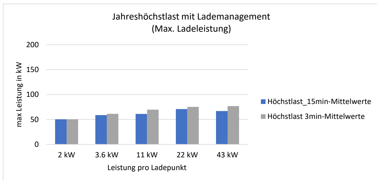
Abbildung 4: Jahreshöchstlasten bei Strategie "Max. Ladeleistung" (mit Lastmanagement)
