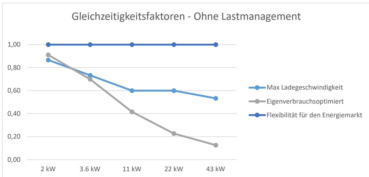
Abbildung 8: Maximale Gleichzeitigkeitsfaktoren bei der Ladeinfrastruktur ohne Lastmanagement
