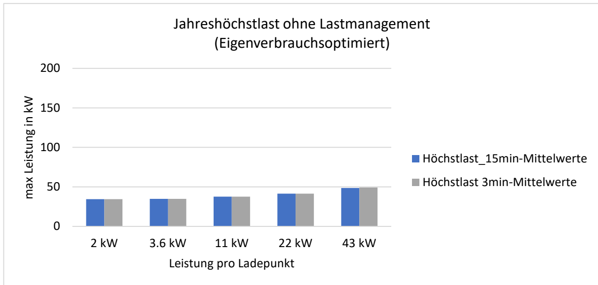
Abbildung 5: Jahreshöchstlasten bei Strategie "Eigenverbrauchsoptimierung" ohne Lastmanagement
