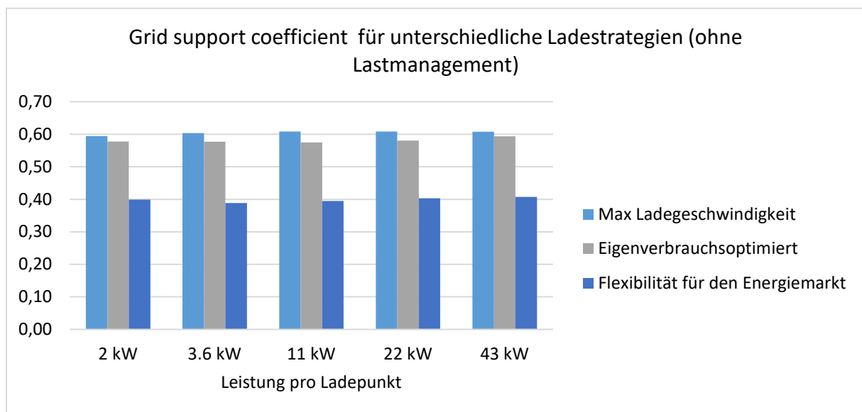
Abbildung 11: Grid support coefficient für die verschiedenen Ladestrategien und Ladeleistungen (ohne Lastmanagement)
