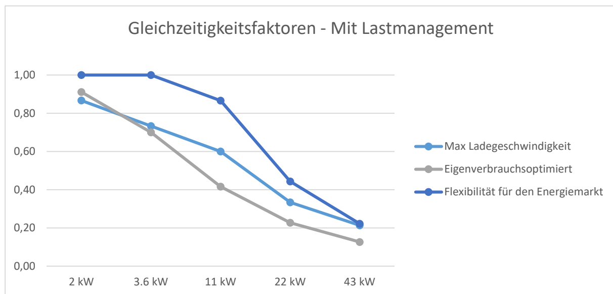
Abbildung 9: Maximale Gleichzeitigkeitsfaktoren bei der Ladeinfrastruktur mit Lastmanagement
