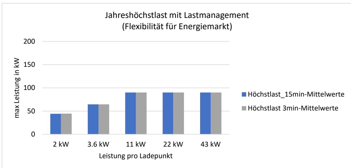
Abbildung 7: Jahreshöchstlast bei Strategie „Flexibilität für Energiemarkt“ mit Lastmanagement
