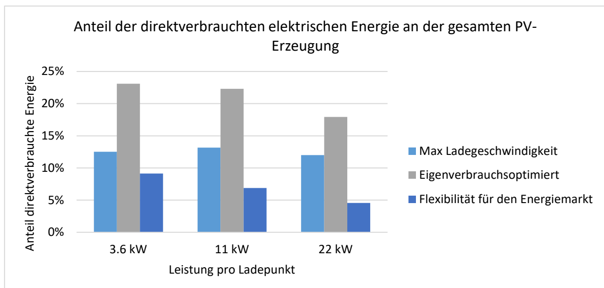
Abbildung 10: Anteile des PV-Stroms für die direkte Ladung der E-Fahrzeuge
