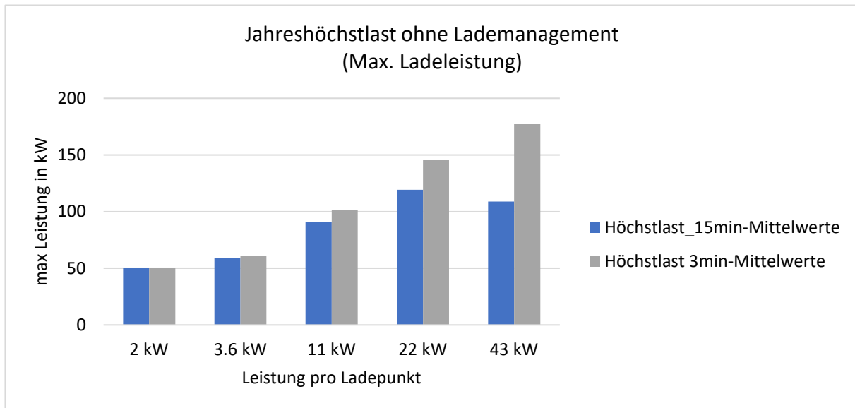
Abbildung 3: Jahreshöchstlasten bei Strategie "Max. Ladeleistung" (ohne Lastmanagement)
